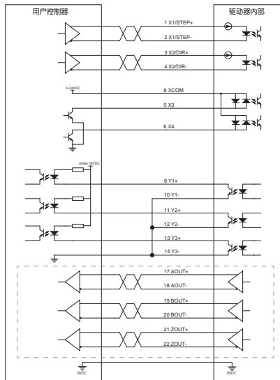
虚线框内编码器输出功能仅P型支持
