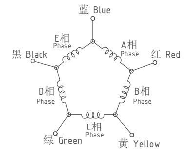
接线图 Wire Diagram
